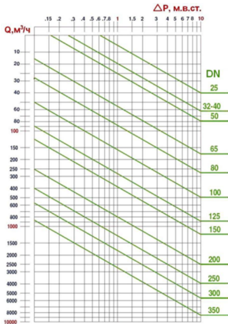
Диаграмма зависимости потерь давления (Среда: вода с температурой T=+20° С)
