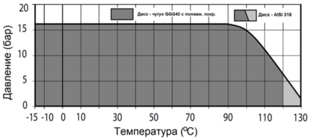
График Температура-Давление
