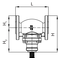
VGF DN 15-25
