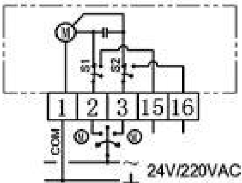
Электрическая схема AMV-1000R
