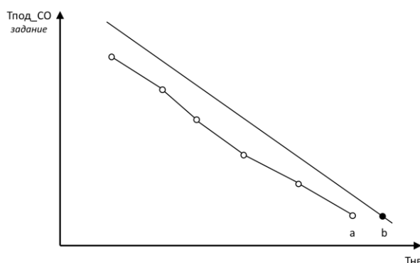
Рис.41. Два варианта задания отопительного графика: график по точкам (а) и через угол наклона (b).
