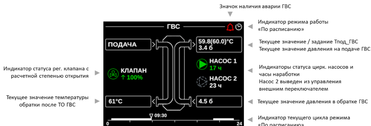
Рис.11. Мнемосхема модуля ГВС.
