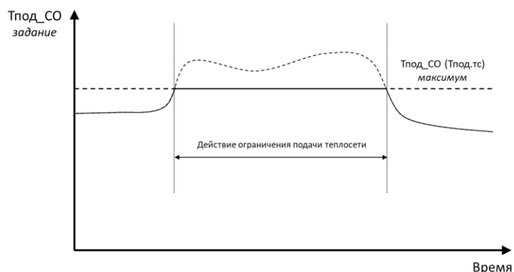
Рис.46. Схема алгоритма ограничения Тпод_СО по температуре подачи теплосети Тпод.тс.
