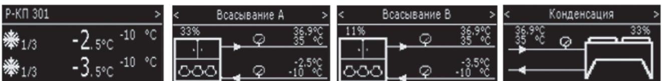
2 группы всасывания и 1 группа конденсатора
