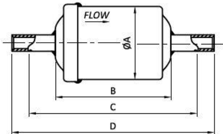
Типоразмер DFL 05-75
