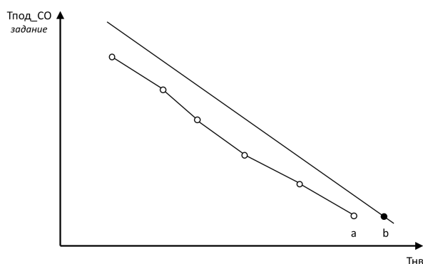
Рис.36. Два варианта задания отопительного графика: график по точкам (а) и через угол наклона (b).
