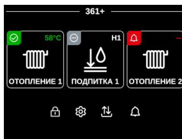
Рис.7. Пример дисплея с модулями автоматики с разными статусами – в работе, остановлен и в аварии.
