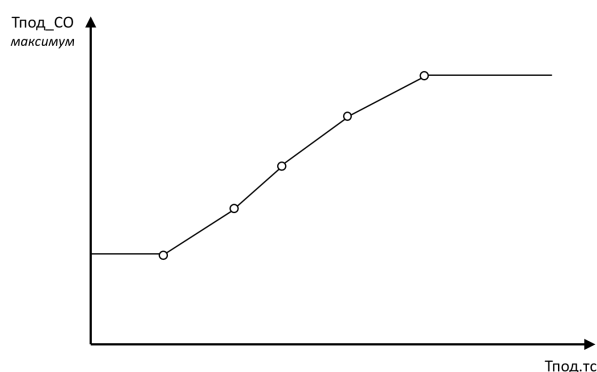
Рис.40. Ограничение температуры подачи в системе отопления от температуры подачи теплосети.
