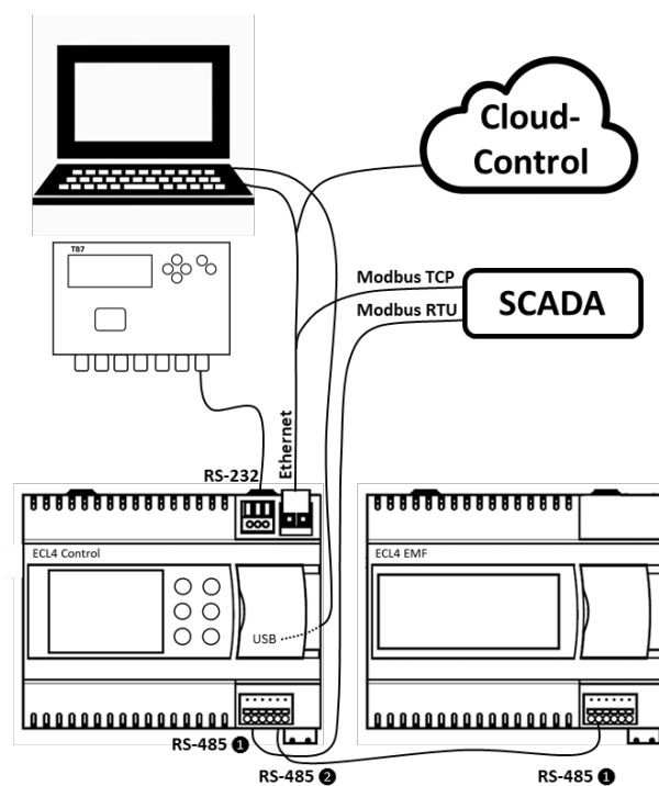
Рис.18. Схема коммуникационных подключений контроллера ECL4 Control 361 Plus Ethernet.
