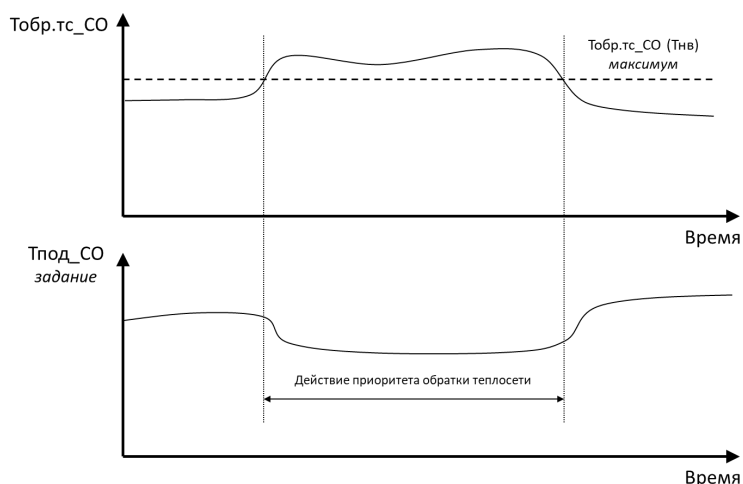
Рис. 39. Схема алгоритма ограничения T_{под\_CO} по обратной температуре теплосети.
