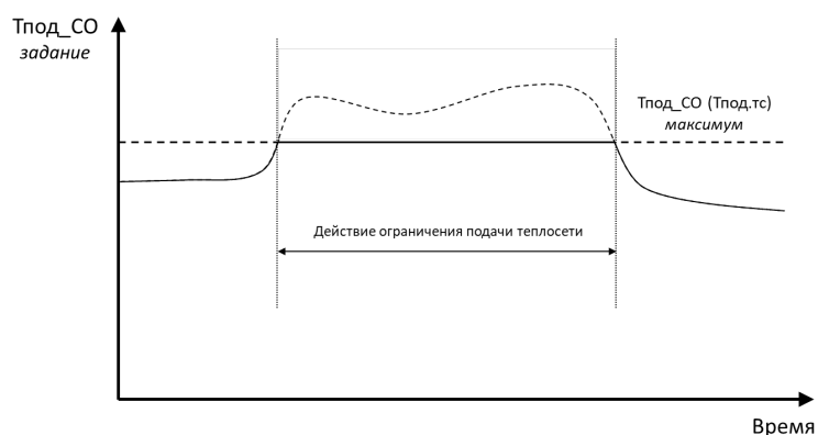
Рис.41. Схема алгоритма ограничения Т под_СО по температуре подачи теплосети Т под.тс .
