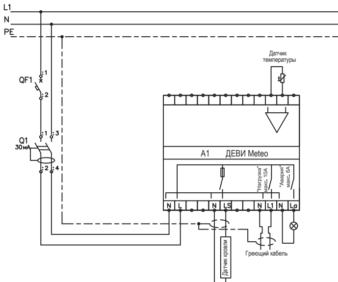
Рис. 14. Схема прямого подключения греющего кабеля
