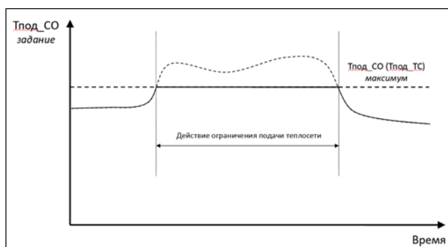
Рис. 8. Схема алгоритма ограничения Т под_СО по температуре подачи теплосети Т под.тс
