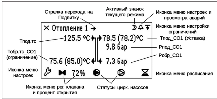
Рис. 21. Экран отопления
