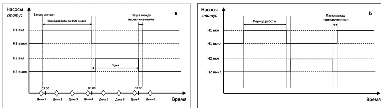
Рис. 11. Схема ротации циркуляционных насосов CO: режимы переключения «по дням» (а) и «по часам» (б). Настройки в примере (а): период = 3 дня, время переключения = 3:00.
