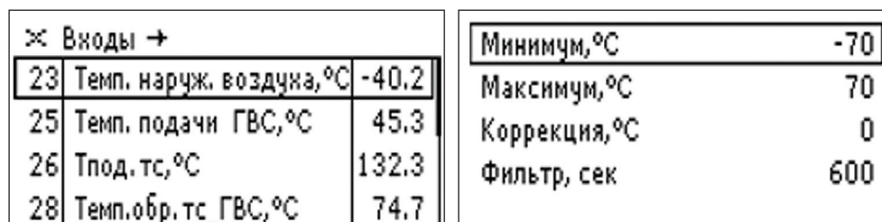
Рис.20. Меню входов-выходов с подменю настройки датчика Тнв.
