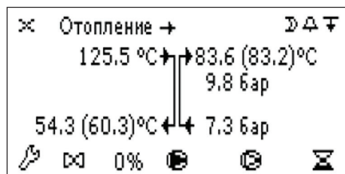
Рис.24. Экран Отопления.
