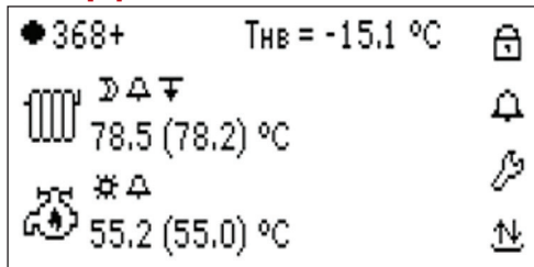
Рис.18. Главный экран.
