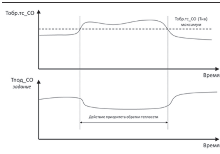
Рис.10. Схема алгоритма ограничения T_{под\_CO} по обратной температуре теплосети.
