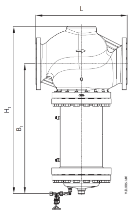
VFGS Ду 150-250 с удлинителем штока
