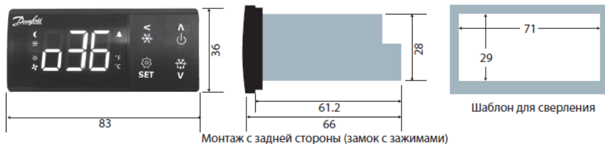
Рис. 2 Габаритные размеры контроллеров температуры типа ERC.
