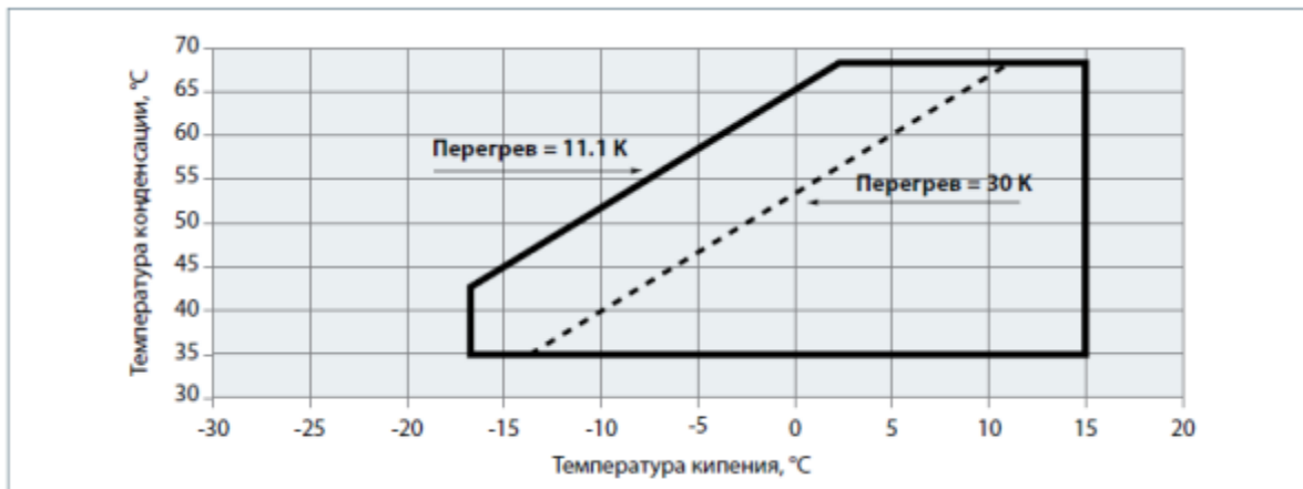
Область эксплуатации компрессоров MTZ с хладагентом R407C (при температуре точки росы)
