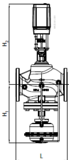
AMV(E) 55/AFQM 2 Ду 65–250, Py 16/25 AMV(E) 56/AFQM 2 Ду 65–125, Py 16/25
