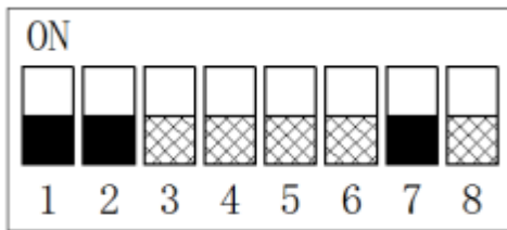
Сигнал управления 4-20мА/Обратная связь 4-20мА
