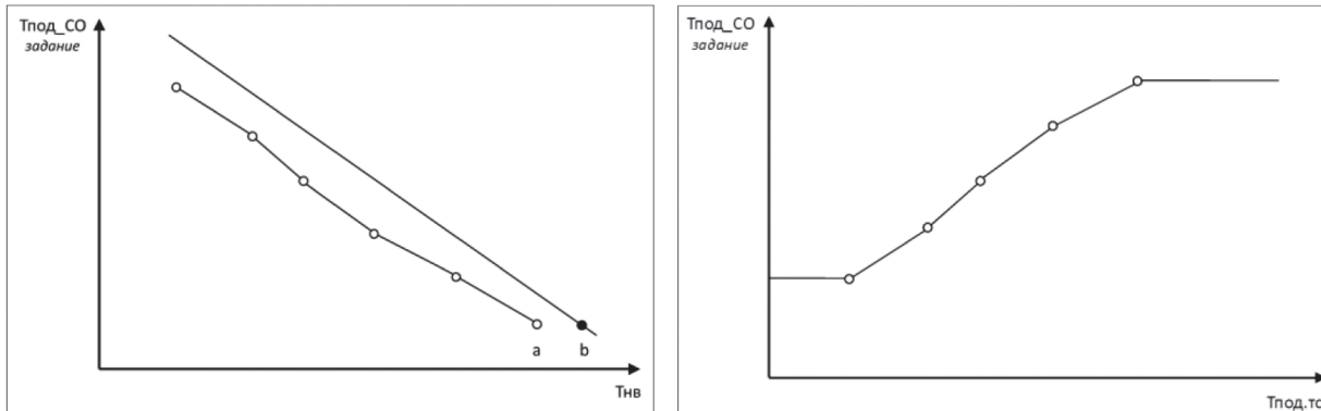
Рис. 8. Два типа регулирования температуры подачи: погодозависимое Tпод (Tнв) с возможностью задания отопительного графика по точкам (a) или через угол наклона (b) и как функция от температуры подачи в теплосети Tпод (Tпод.тс).
