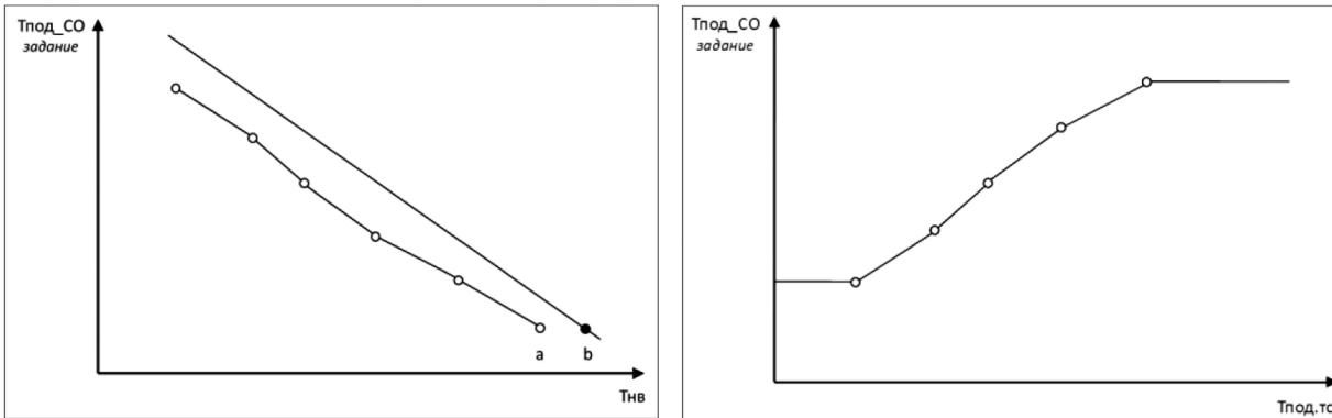
Рис. 8. Два типа регулирования температуры подачи: погодозависимое Тпод (Тнв) с возможностью задания отопительного графика по точкам (а) или через угол наклона (b) и как функция от температуры подачи в теплосети Тпод (Тпод.тс).
