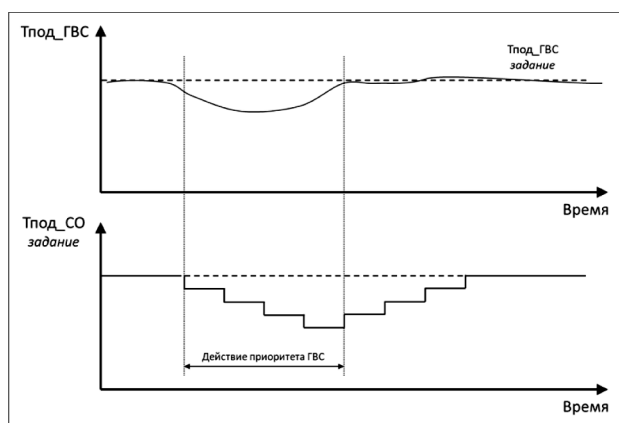
Рис. 3. Схема алгоритма ограничения Т под_СО по приоритету ГВС
