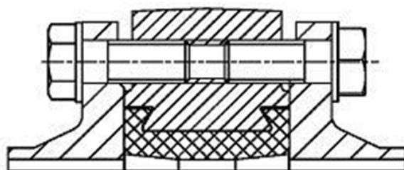
В резьбовые отверстия корпуса
