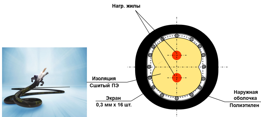
Рис. 2. Устройство нагревательного кабеля DEVIaqua™ 9T.
