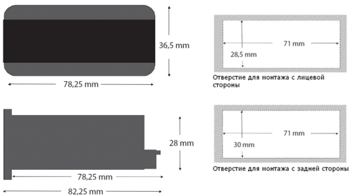
Рис. 2 Габаритные размеры контроллеров температуры типа ERC.
