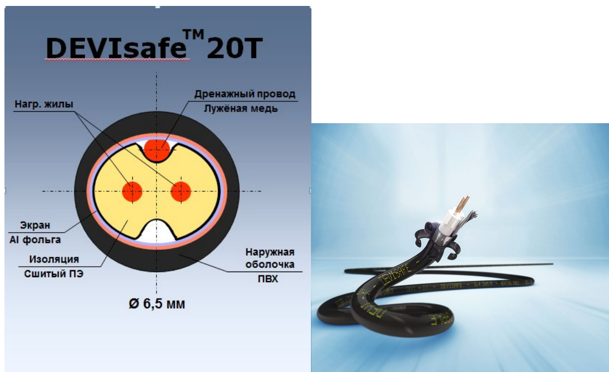
Рис. 2. Устройство нагревательного кабеля DEVIsafe™ 20T .
