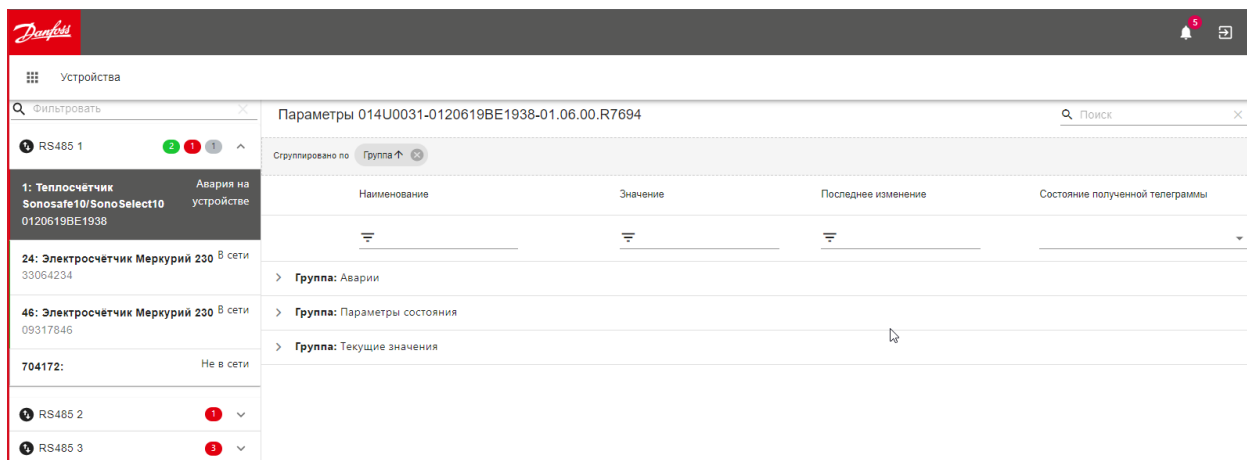
Рис. 6. Страница «Устройства»
