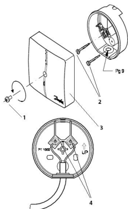
Устройство датчика температуры типа ESMT
