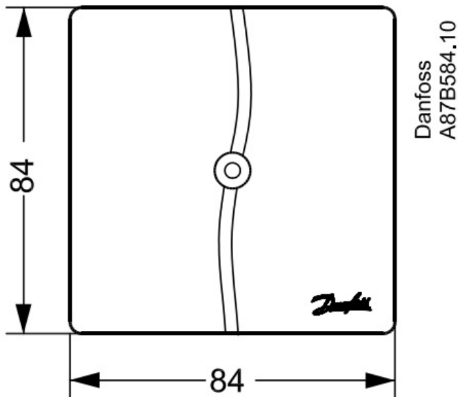
Габаритные размеры датчика температуры типа ESMT
