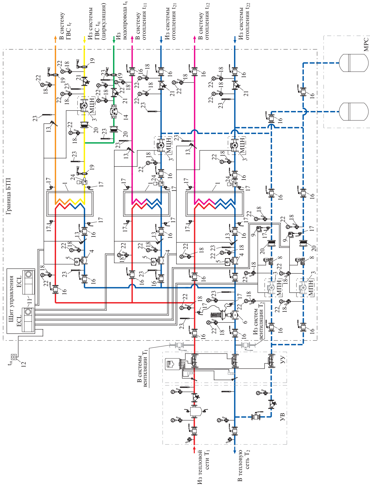
Рис. 8. Технологическая схема № 7 БТП для двух систем отопления при независимом присоединении к тепловой сети и системы ГВС с одноступенчатым водоподогревателем.
