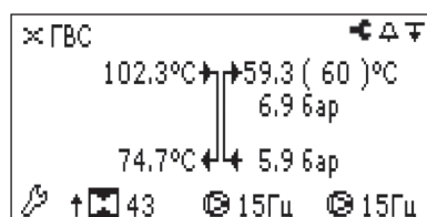
Рис. 12. Пример управления рег. клапаном ГВС в Ручном режиме.
