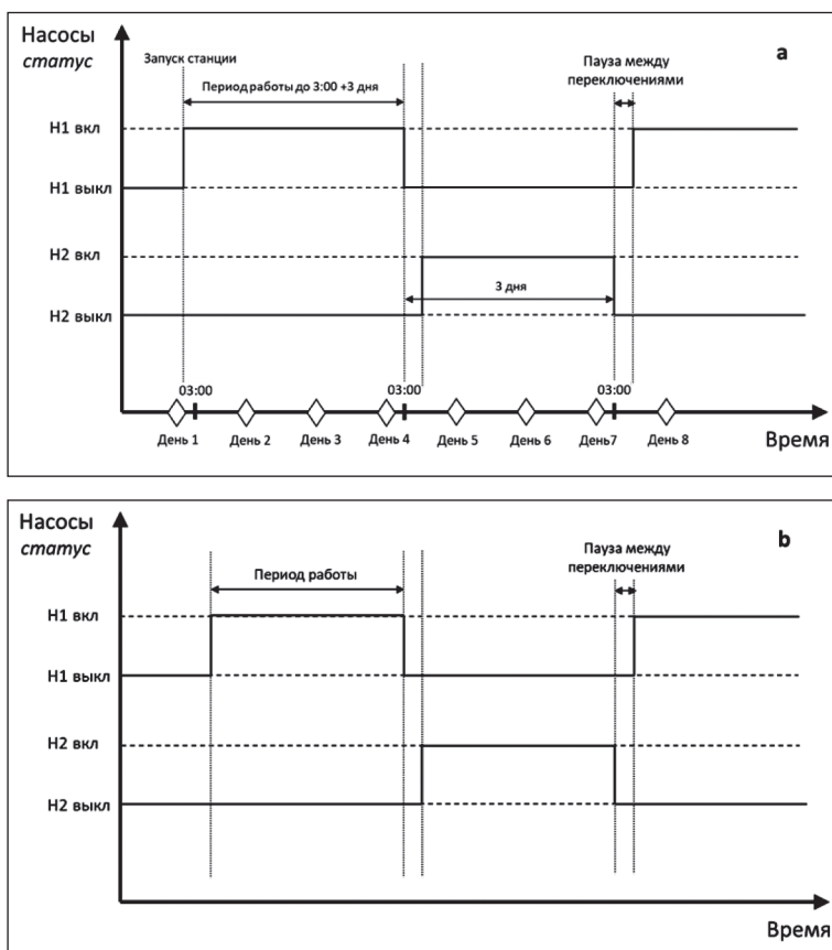
Рис. 3. Схема ротации циркуляционных насосов ГВС: Режимы переключения «по дням» (а) и «по часам» (б). Настройки в примере (а): Период = 3 дня, время переключения = 3:00.
