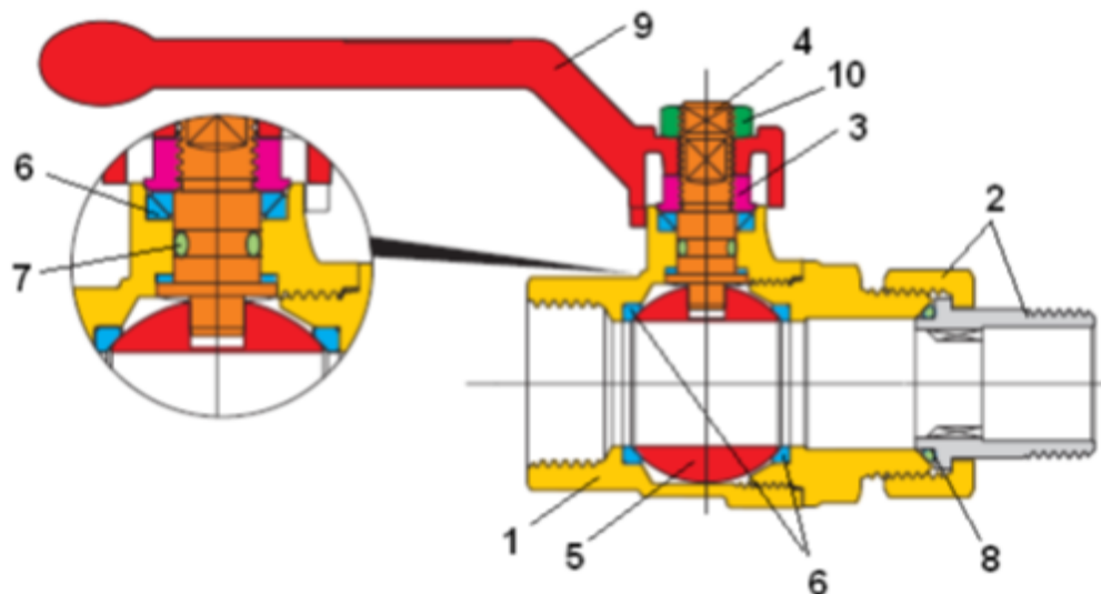
рис.2: Материалы деталей крана DN 32 мм.
