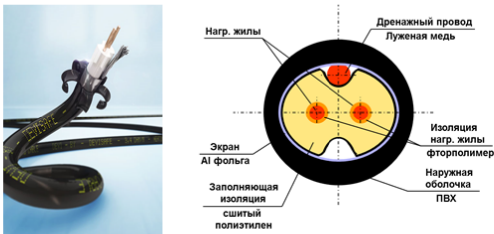
А) В) Рис. 2. Устройство нагревательного кабеля DEVIsnow™ 30T.
