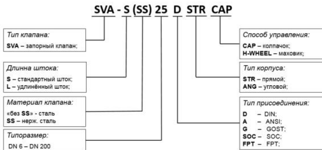
Рис. 3 Пример схемы обозначения клапанов SVA
