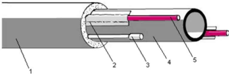
Рис. 4. Монтаж нагревательного кабеля DEVIflex™ 10T на водопроводных трубах.
