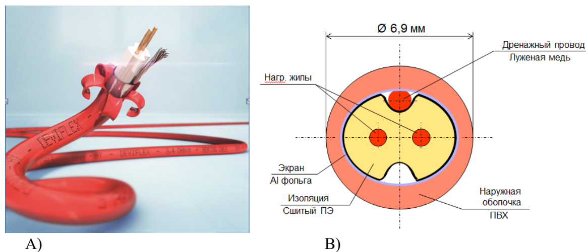
Рис. 2. Устройство нагревательного кабеля DEVIflex™ 10T.
