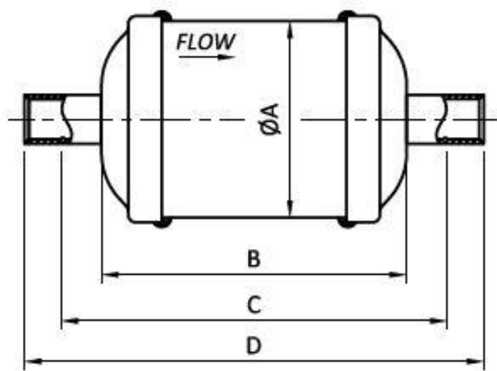
Типоразмер DFL 05-75
