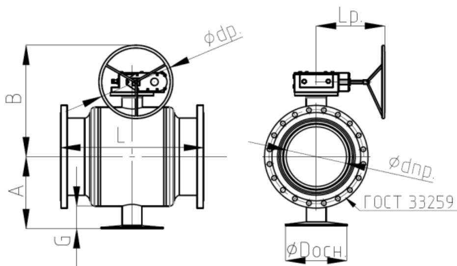
Габаритные и присоединительные размеры кранов шаровых типа RJP в мм.
