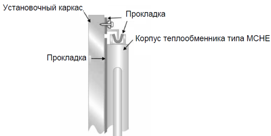
Монтаж теплообменников микроканальных типа МСН.
