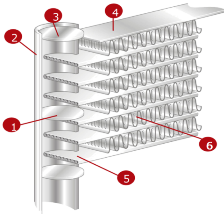
Устройство теплообменников микроканальных типа МСНЕ.
