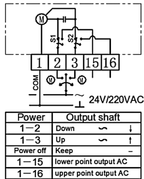
Электрическая схема AMV-1800R
