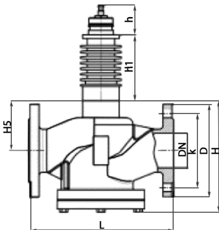
Рис. 2 - Габаритно-присоединительные размеры
