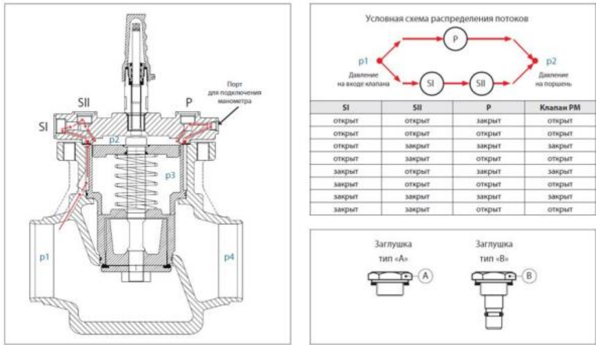
Рисунок 3. Принцип работы
