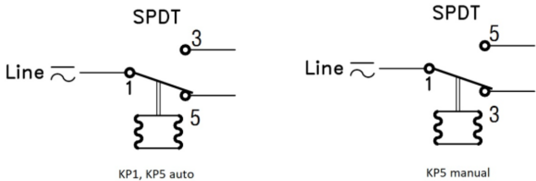
Однополюсная двухпозиционная контактная группа SPDT
