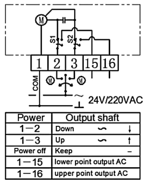
Электрическая схема AMV-1800R
