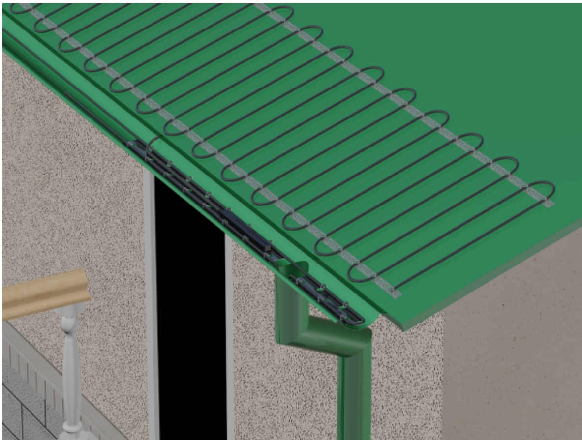
Обогрев капельника карниза с применением двойной монтажной ленты:
