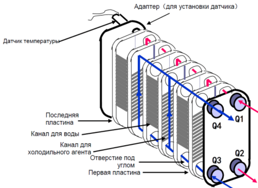
Рис.3 - Схема теплообменника пластинчатого типа BPHE.
