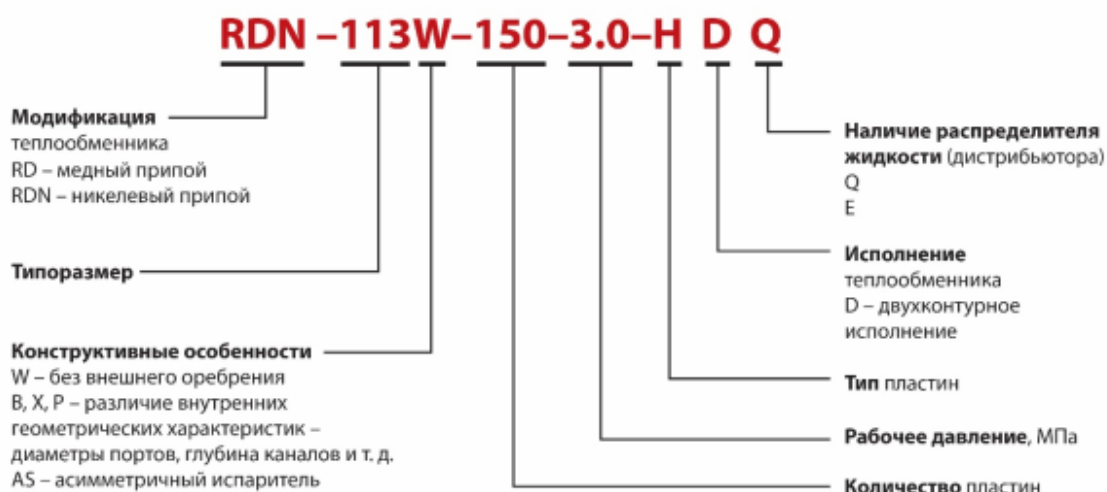
Рис.4 - Пример условного обозначения теплообменников пластинчатых типа BPHE
