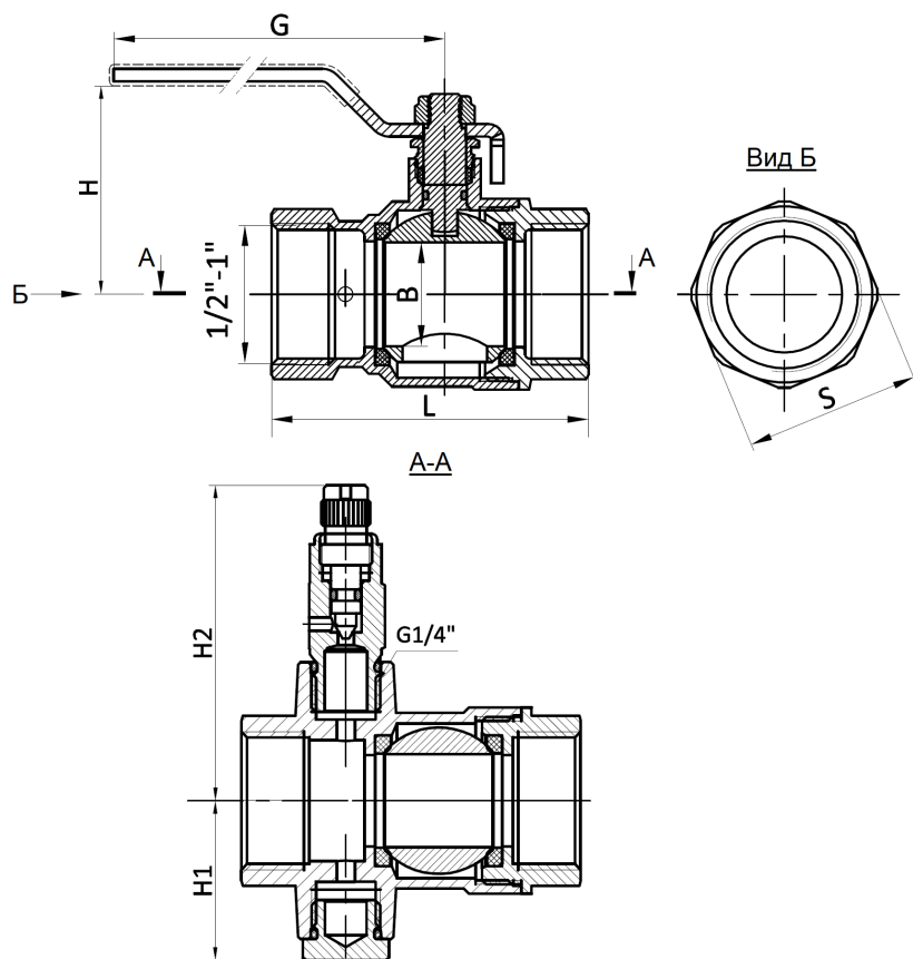
рис.3: Габаритные и присоединительные размеры
