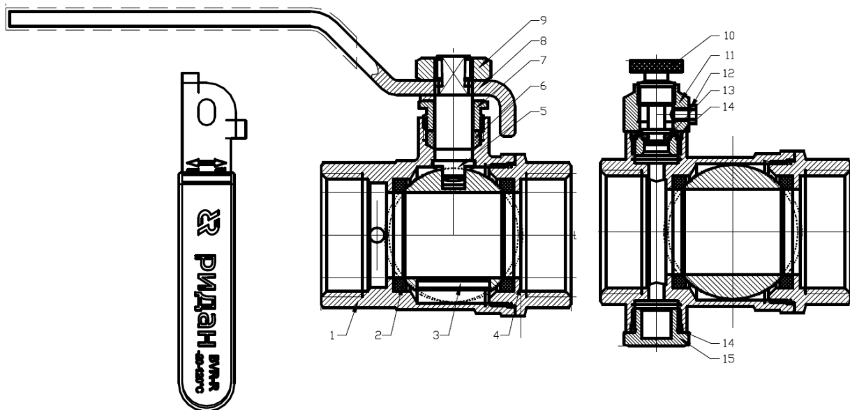
Рис.1 Конструкция шарового крана DN 15-50 мм
