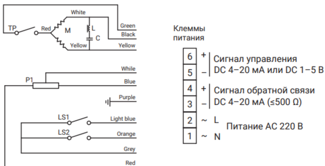
Электрическая схема AME-26KSR
