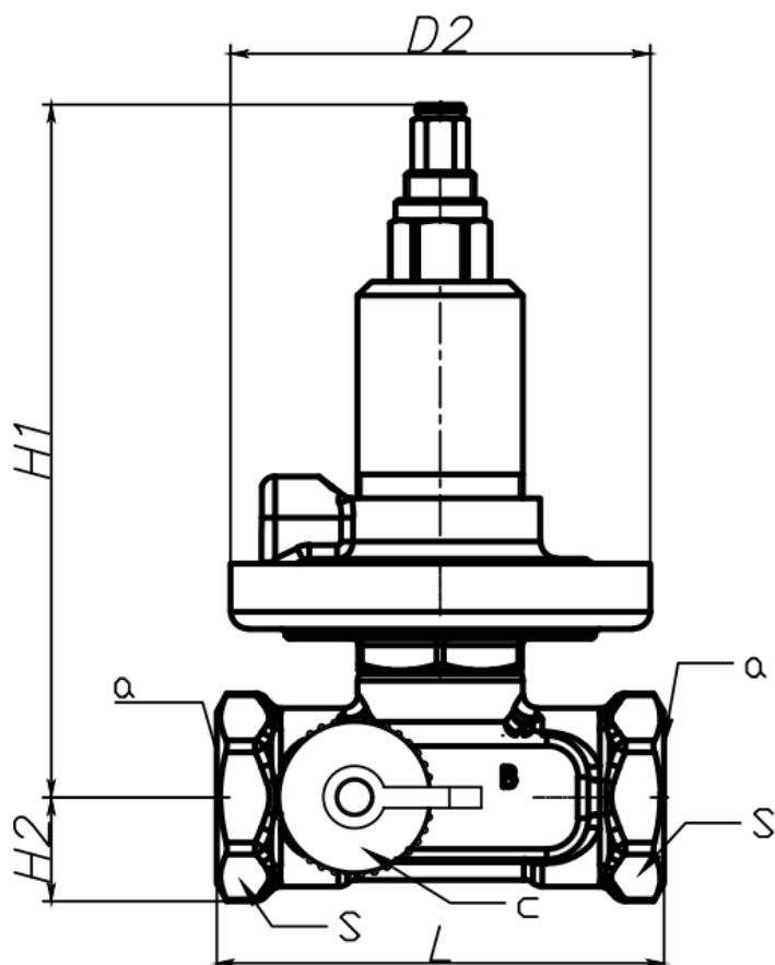
Рис. 3. Габаритные и присоединительные размеры клапанов АРТ-R3 DN=15 – 25 мм.
