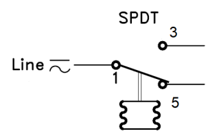
Рис.3.2. Контактная система
