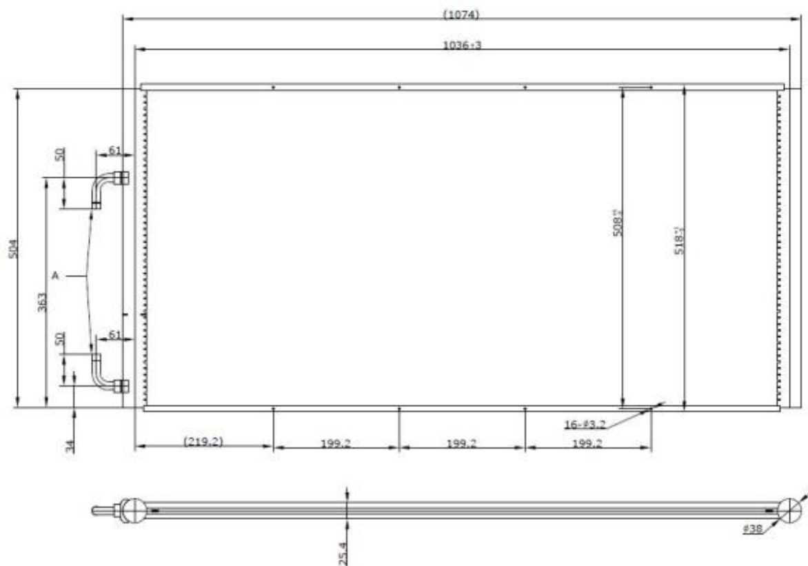
Габаритные размеры и изображение теплообменника микроканального модификации RC-1500.
