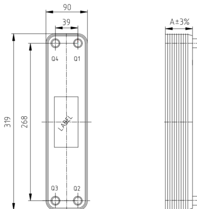
Рис.6 - Габаритные размеры и изображение теплообменника пластинчатого модификации BPHE_RD-030
