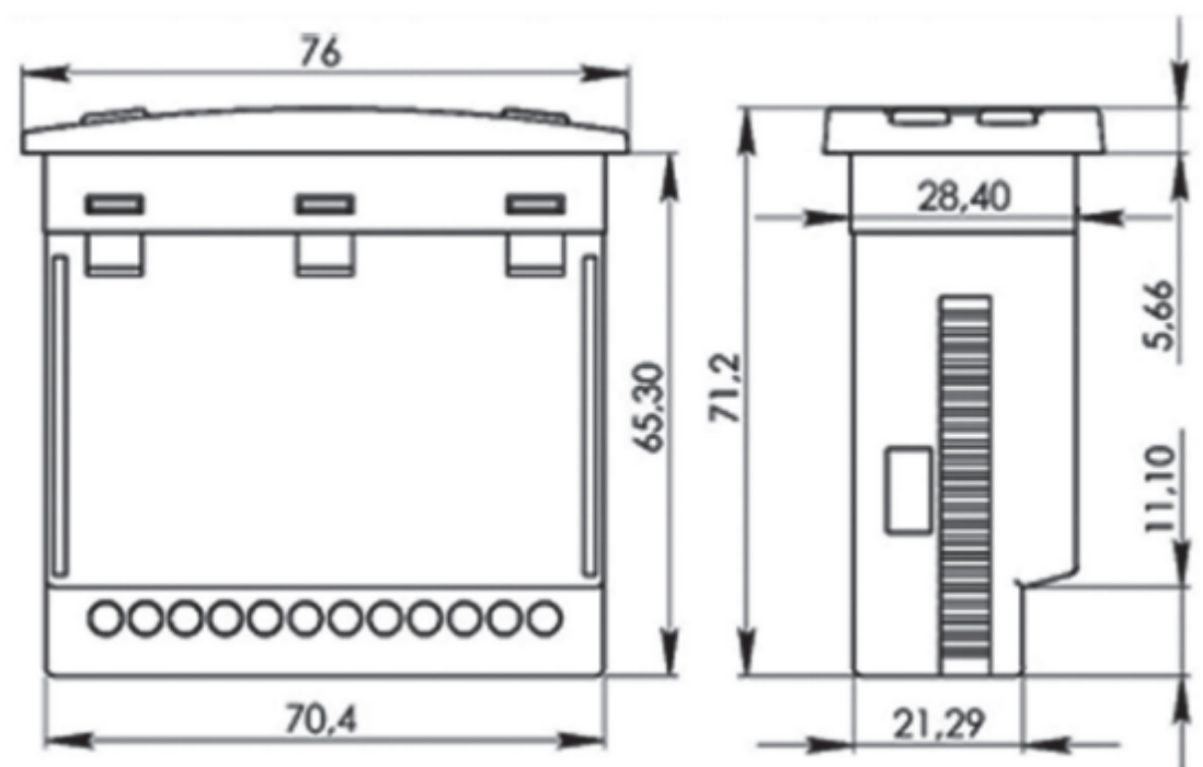
Рис. 2 Габаритные размеры контроллеров Р-КИ 130
